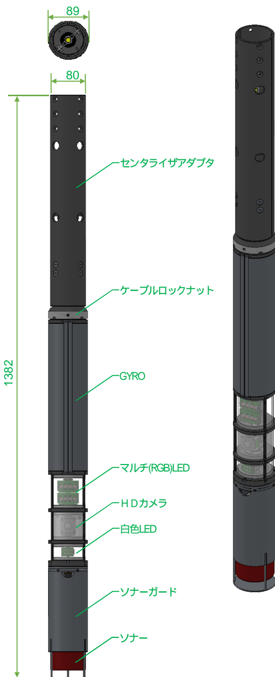
測定管 (ゾンデ) 外形図
